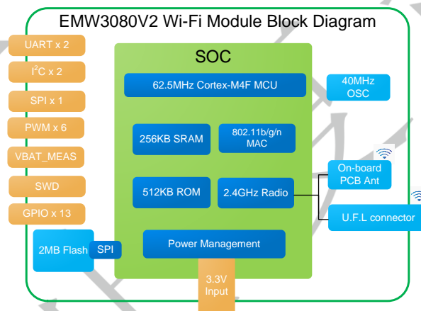
EMW3080V2 硬件框图
