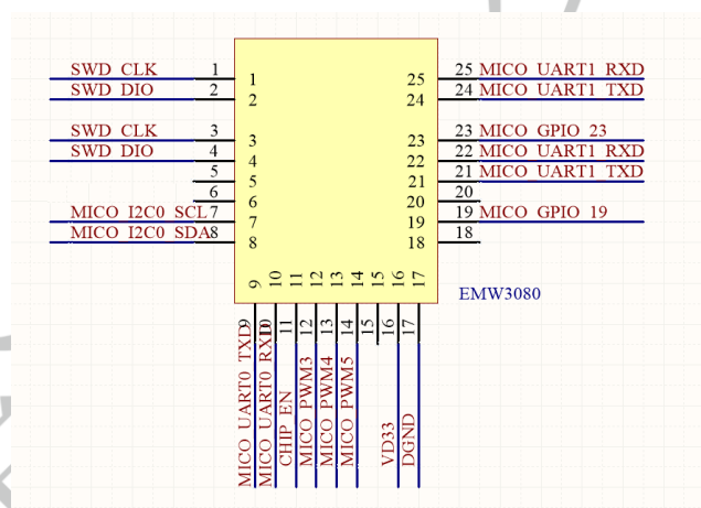
图 13 EMW3080V2 外部接口参考设计
