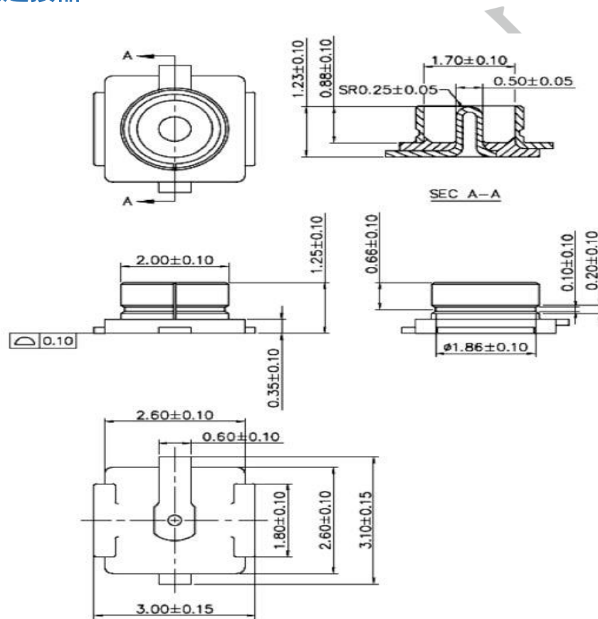
图 6 外接天线连接器尺寸图
