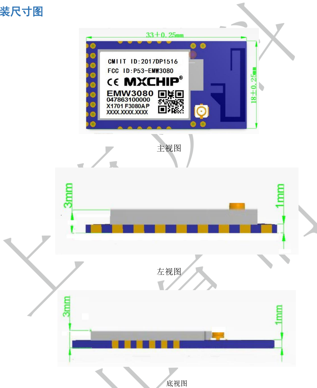
图 7 EMW3080V2 三视图（单位：mm）
