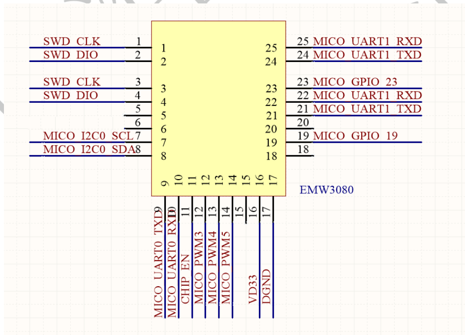
图 4 EMW3080V2 封装定义图
