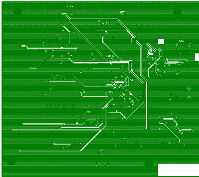
02 - Layer 2
