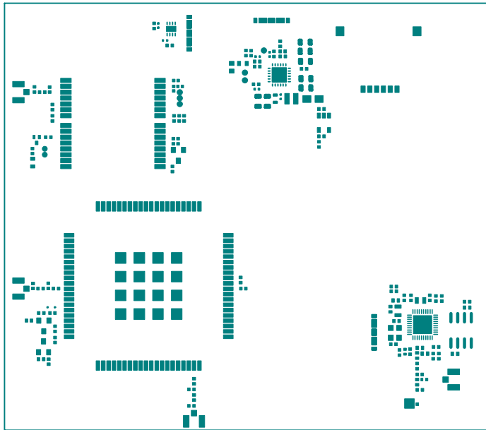
08-Paste Mask Bottom
