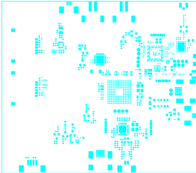
07-Paste Mask Top
