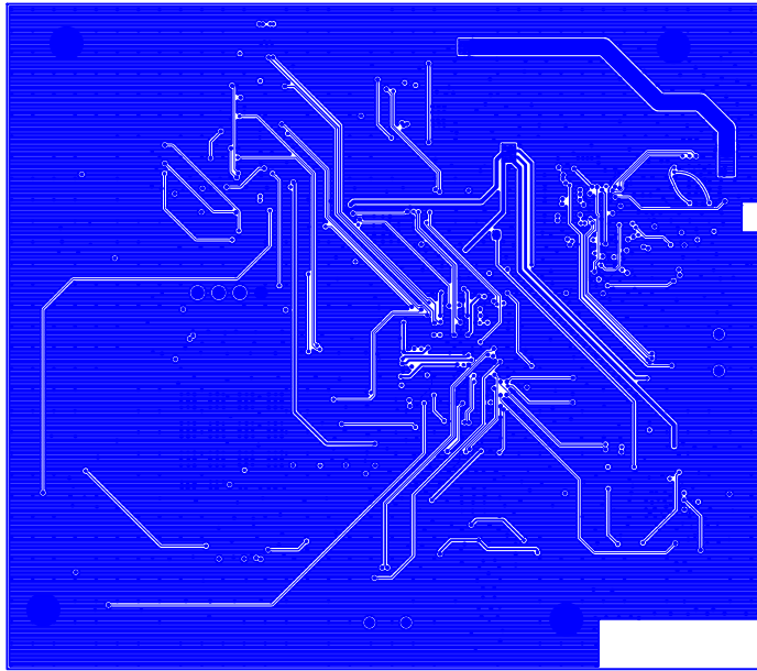
03 - Layer 3
